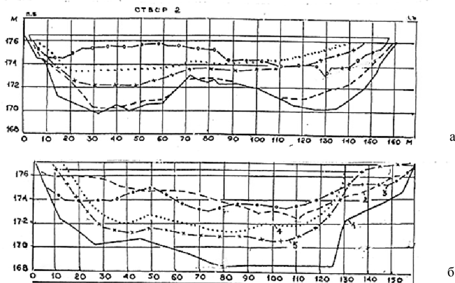
Рис. 1. Совмещенные поперечные профили левобережного (а) и правобережного (б) отстойников Тахиаташского гидроузла: 1 — 1977 г., 2 — 1978 г., 3 — 1979 г., 4 — 1996 г., 5 — 1998 г.
